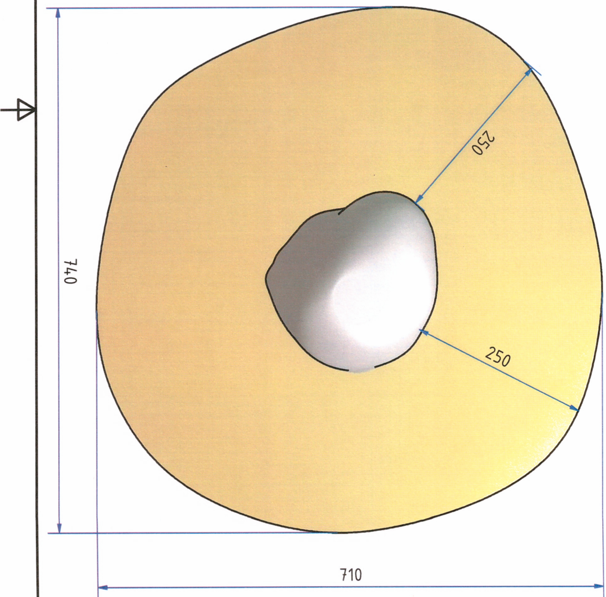
Půdorys dopadiště
